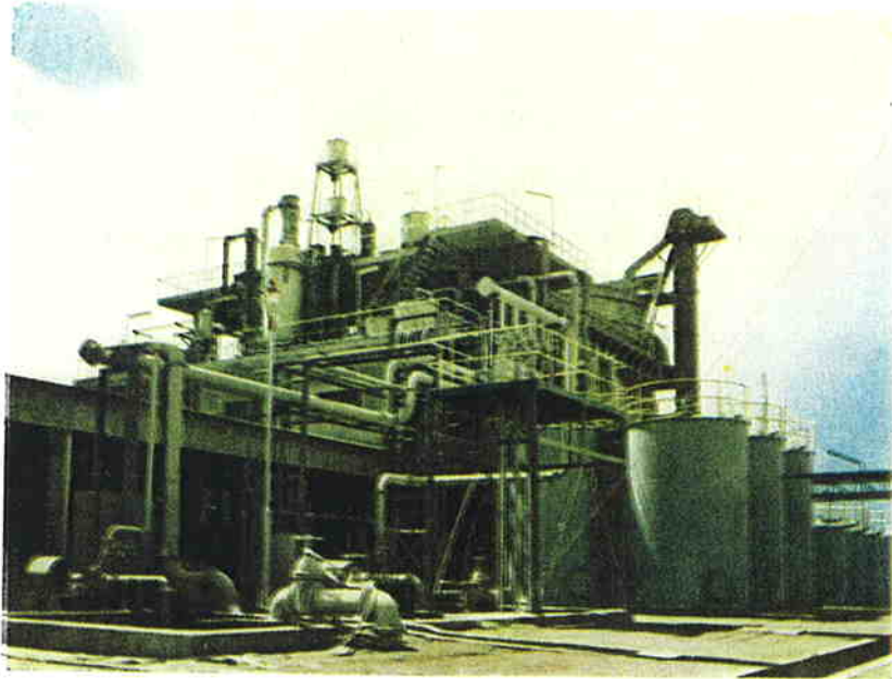
写真 上は 新設のアンモニア工場 下は 建設中のりん酸工場
