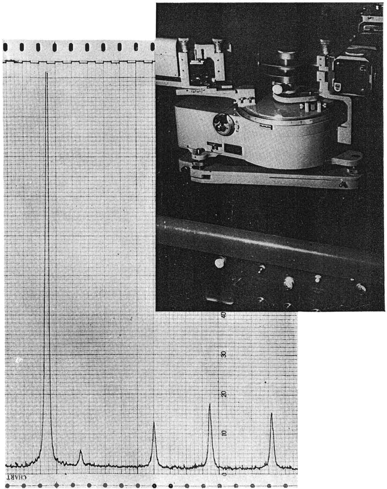
石灰石 X-Ray 回折图形
