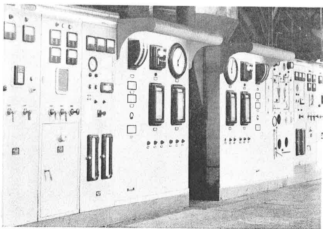
当社セメント工場のロングキルン(上) 並びに制御盤(下)
